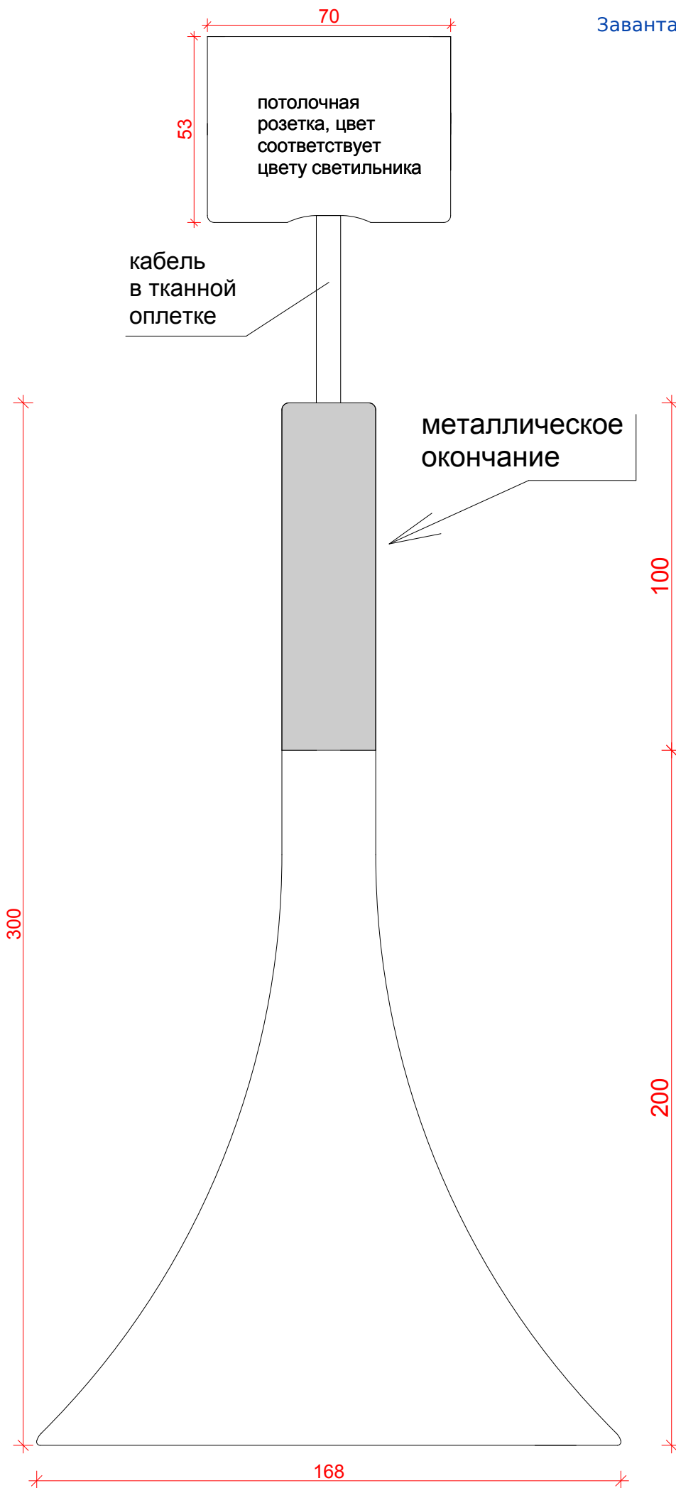
бетонный светильник "ЛЕЙКА"
