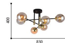
6718-46 ∅ 830 ↑↓ 400 ⚡ E27 220V 6 x 40W IP20 metal, glass
