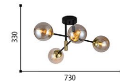
6718-44 ∅ 730 ↑↓ 330 ⚡ E27 220V 4 x 40W IP20 metal, glass
