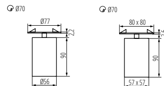
CHIRO GU10 DTO
