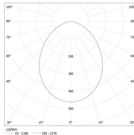
KANLUX S.A. (kat 23362) OMERIS N LED 25W-NW-W / Krzywa rozsyłu światła (biegunowo)
