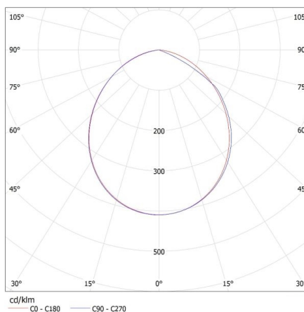
KANLUX S.A. (kat 23550) SEVIA LED 26 / Krzywa rozsytu światła (biegunowo)
