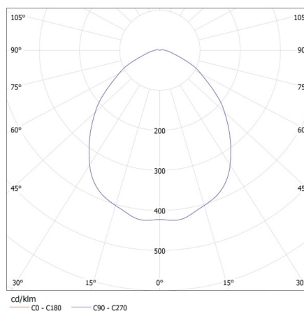
KANLUX S.A. (kat 24430) RANVI LED EL-10 / Krzywa rozsyłu światła (biegunowo)
