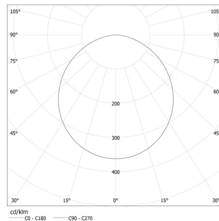
KANLUX S.A. (kat 25562) LITEN LED 8W-WW / Krzywa rozsyłu światła (biegunowo)
