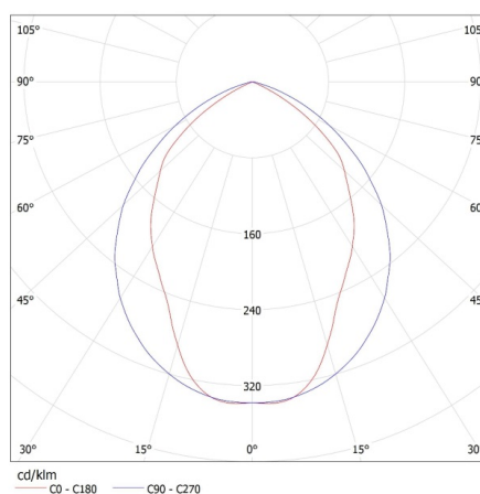
KANLUX S.A. (kat 25710) REGIS 3WS EVG 418 PT / Krzywa rozsyłu światła (biegunowo)
