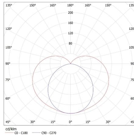
KANLUX S.A. (kat 27531) PESSA LED IP44 9W-NW / LDC (Polar)
