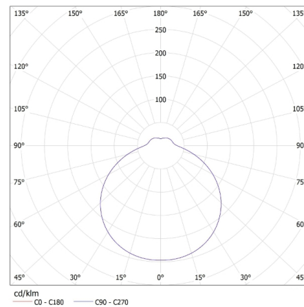
KANLUX S.A. (kat 28723) BIGGE LED 42W-NW-L / LDC (Polar)
