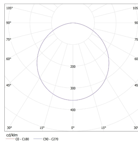
MILEDO (kat 31076) SP LED N 6W WW-R / LDC (Polar)
