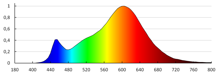
MILEDO (kat 31076) SP LED N 6W WW-R / LDC (Polar)
