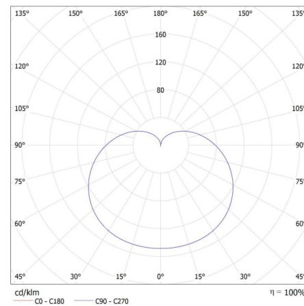
KANLUX S.A. (kat 33716) IQ-LED A60 9,6W-WW / LDC (Polar) Luminaire: KANLUX S.A. (kat 33716) IQ-LED A60 9,6W-WW Lamps: 1 x IQ-LED A60 9,6W-WW
