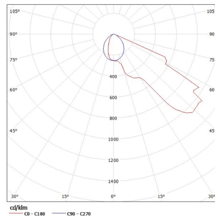
KANLUX S.A. (kat 4684) LICA LED-J04A / Krzywa rozsyłu światła (biegunowo)
