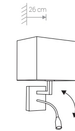
HOTEL LED abażur, stal chromowana / shade, electroplated steel / абажур, хромированная сталь 6800 ● EC 9302 ● GY Ⓛ 1×E27, max 60W, 1×LED 2,2W
