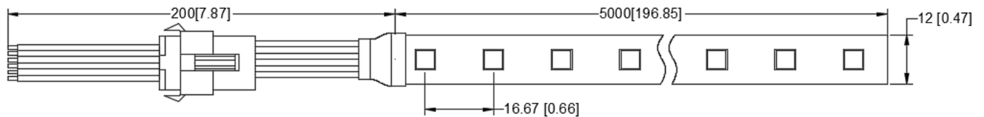
RD6260AC-A
