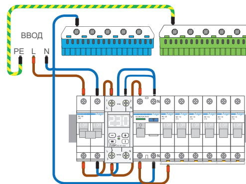
Схема 4. Варіант монтажною схеми без транзиту нуля через D2
