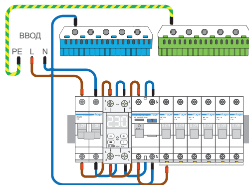
Схема 2. Варіант монтажною схеми з транзитом нуля через D2
